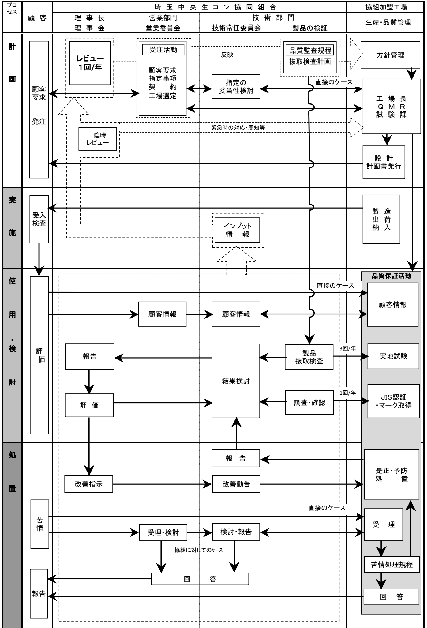
図1 埼玉中央生コン協同組合品質保証体系図
